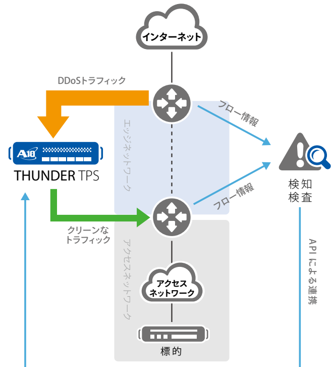
アシンメトリックモードのTPS
