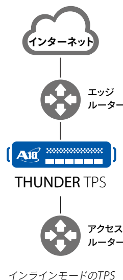
インラインモードのTPS
