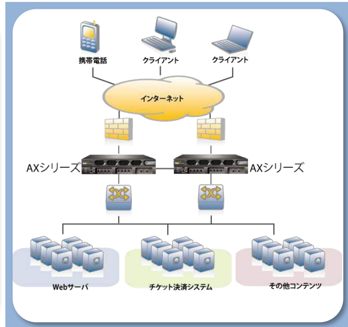
チケットWeb松竹 構成図
