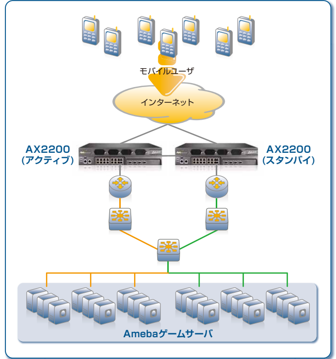
Amebaゲームネットワーク構成図
