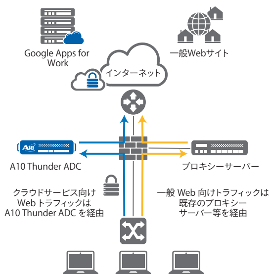
図1: クラウド向けのWebトラフィックをA10 Thunder ADCに集約
