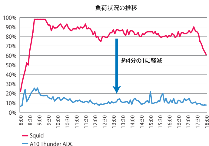
図2: A10 Thunder ADCの導入後、プロキシにかかる負荷が業務時間を通じて大幅に低減
